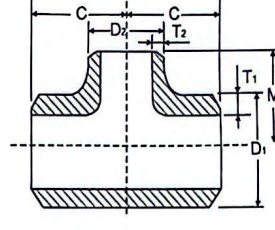
对焊异径三通 BW Reducing Tee
