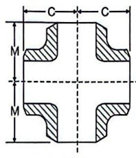
对焊等径四通 BW Straight Cross
