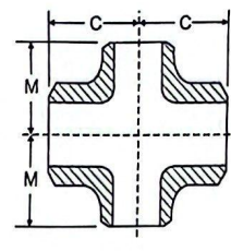
对焊异径四通 BW Reducing Cross
