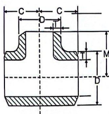
对焊等径三通 BW Straight Tee
