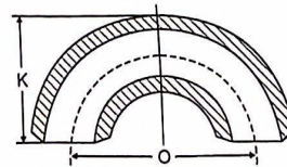
对焊180° 长半径/短半径弯头 BW180° Return LR/SR
