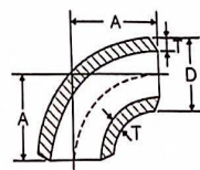
对焊90° 长半径/短半径弯头 BW90° Elbow LR/SR
