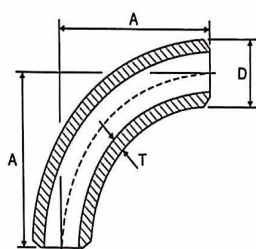
对焊90° 3D、5D、10D弯头 BW90° 3D、5D、10D Elbow
